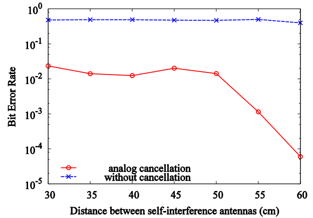
그림 2. 송수신 안테나 거리에 따른 BER
