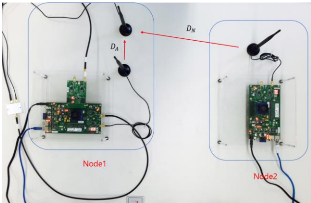
그림 1. WARP SDR 보드로 구현한 전이중 통신 실험환경
